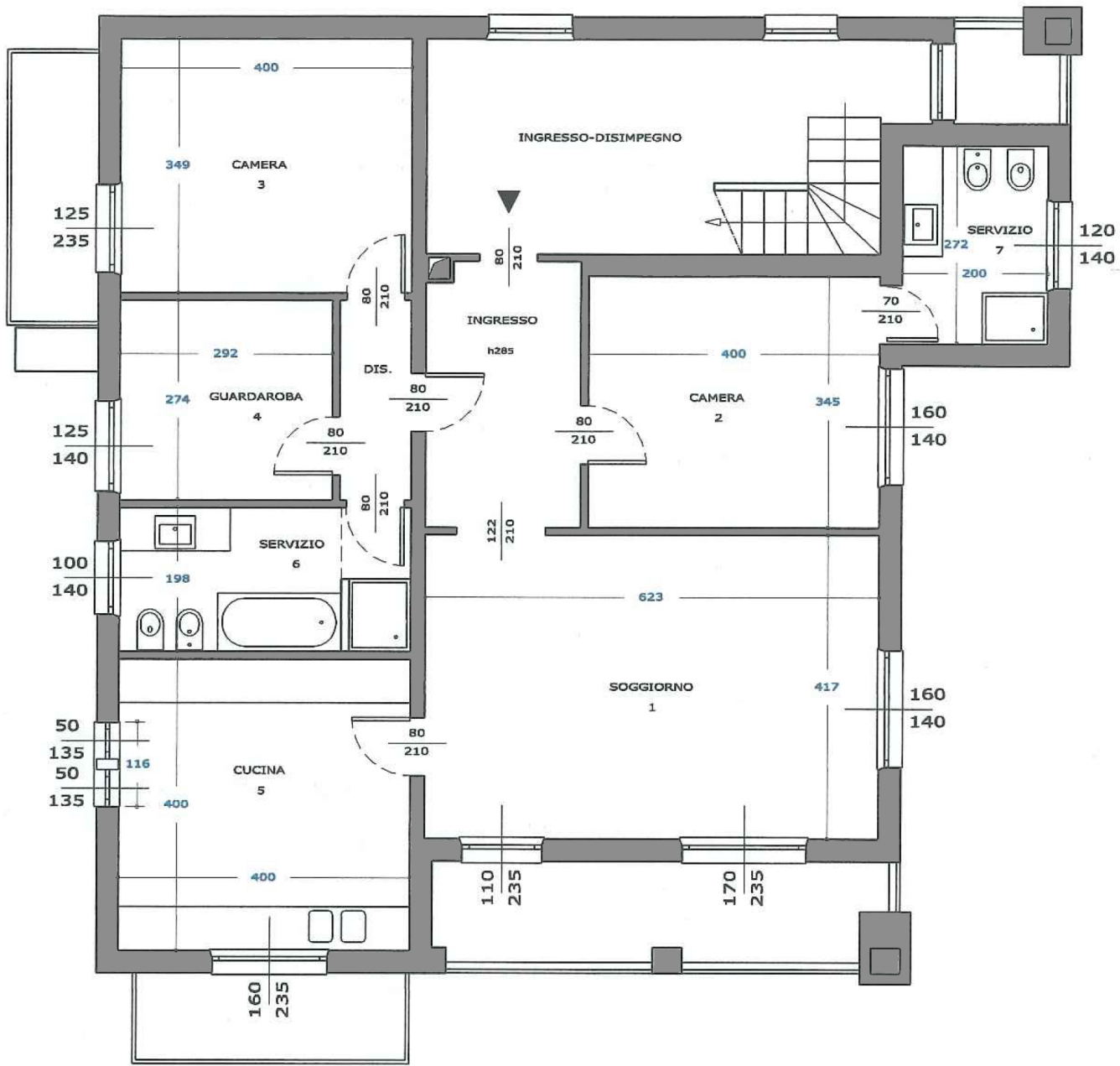
PIANO PRIMO
