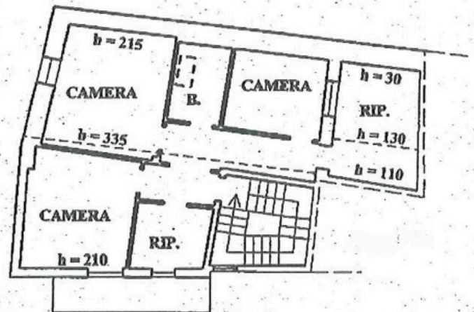
SECONDO PIANO
