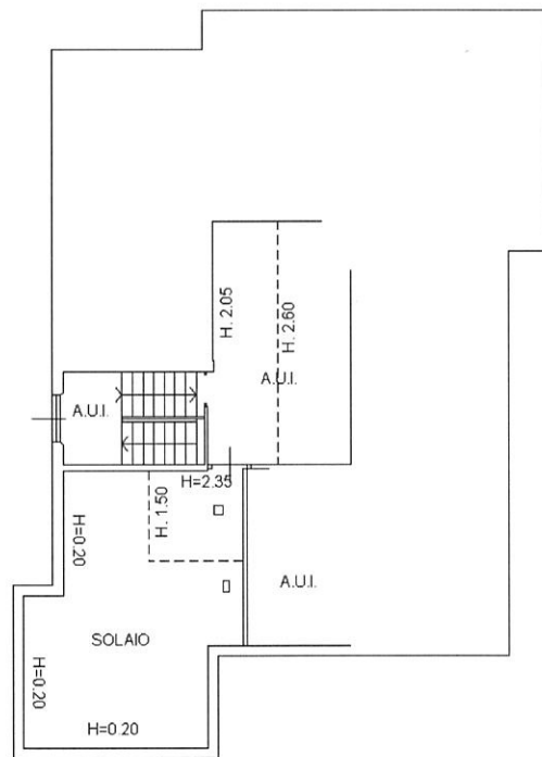
PIANO TERZO
