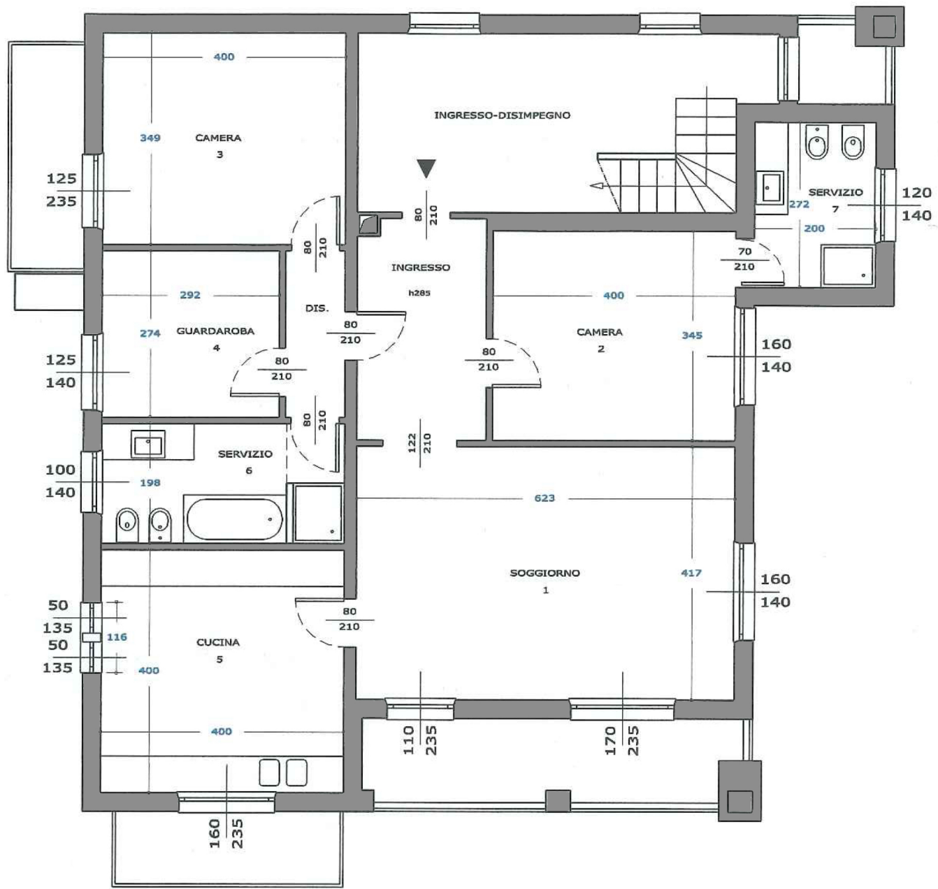
PIANO PRIMO
